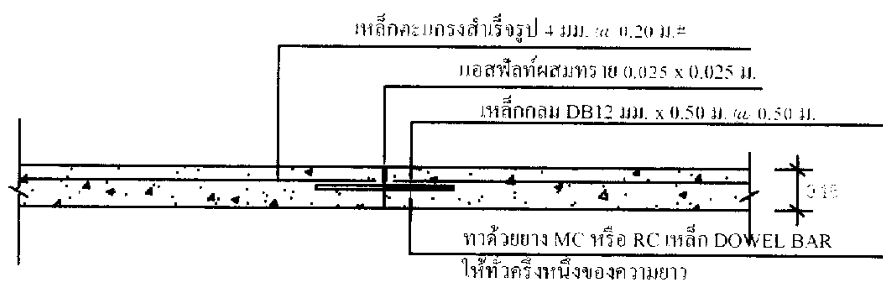
แบบขยายรอยต่อ CONSTRUCTION JOINT
